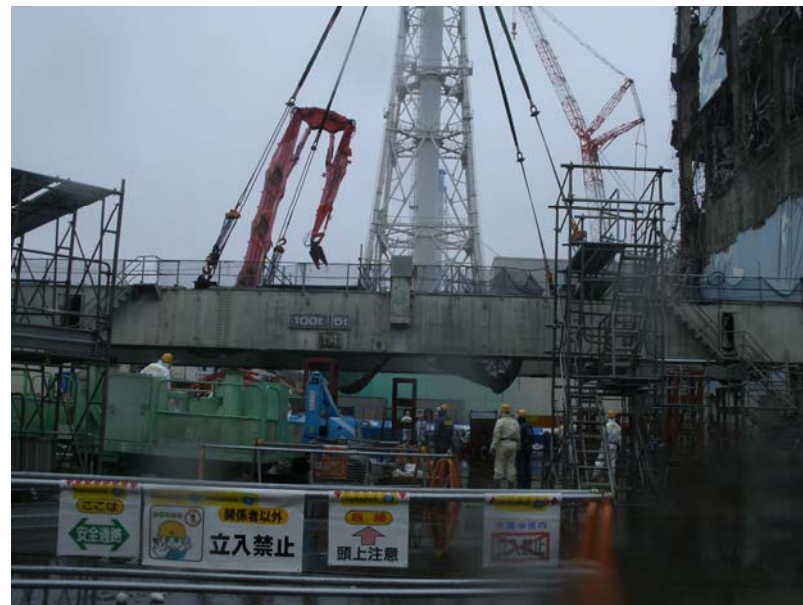
⑧ 天井クレーンガーダー撤去作業(4)
