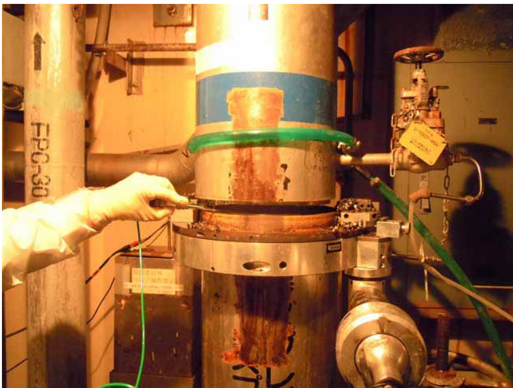
< 配管下部切断後 >
