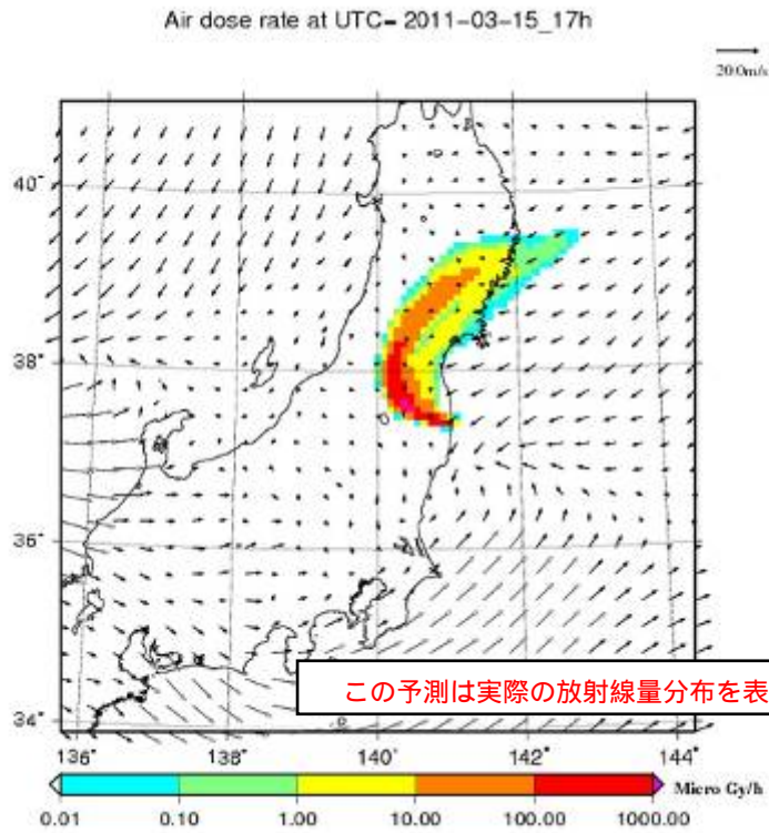
【空間線量率分布 3月16日 4時】
