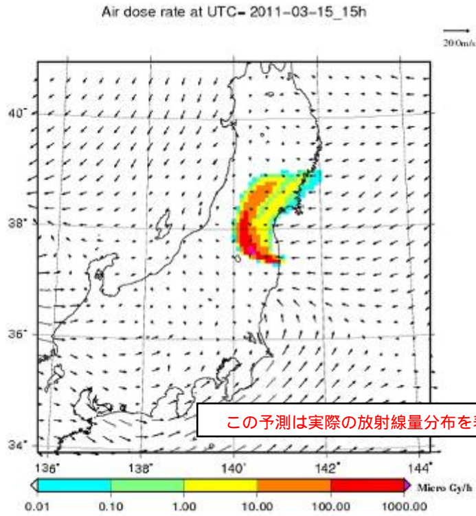
【空間線量率分布 3月16日 2時】
